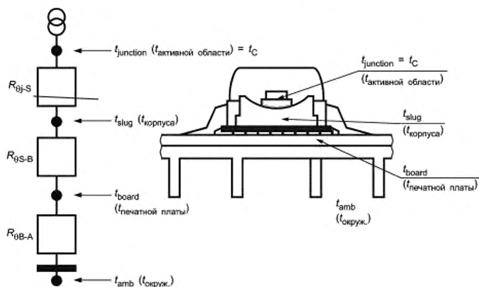
Рисунок 1 — Схематическая цепочка тепловых сопротивлений
