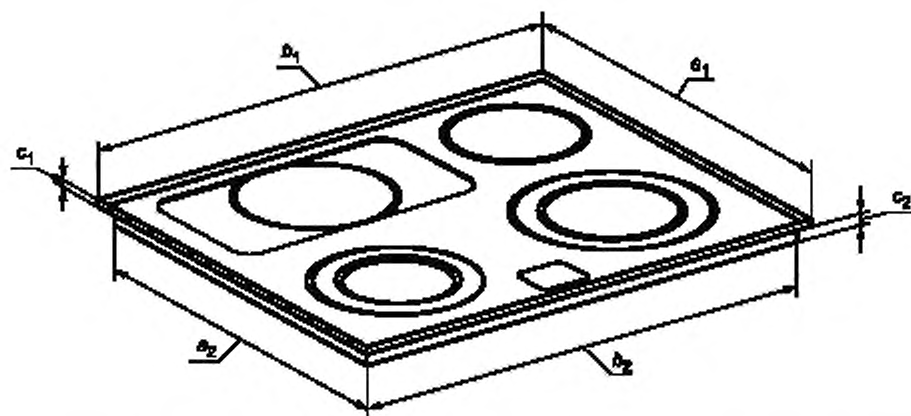
Рисунок 2 — Размеры для встроенных жарочных шкафов
