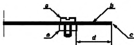
Рисунок 11 — Расположение термопары для измерения температуры окружающей среды
