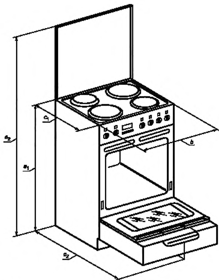
Рисунок 1 — Размеры приборов
