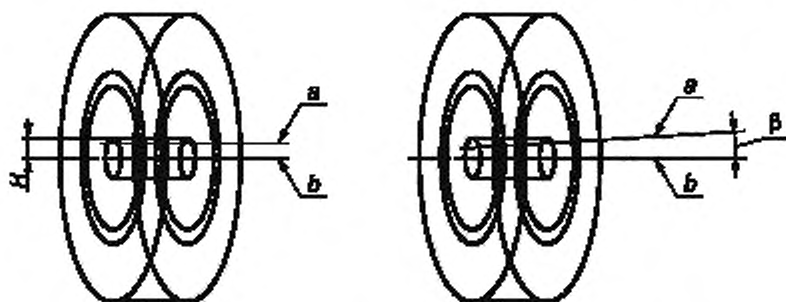
Рисунок 1 — Отклонение линии действия нагрузки от оси подшипника
