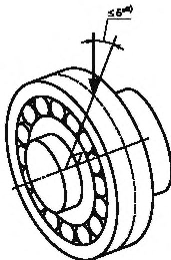
Рисунок 3 — Отклонение от радиальной оси (ИСО 15242-3:2006/Попр.1:2010)
