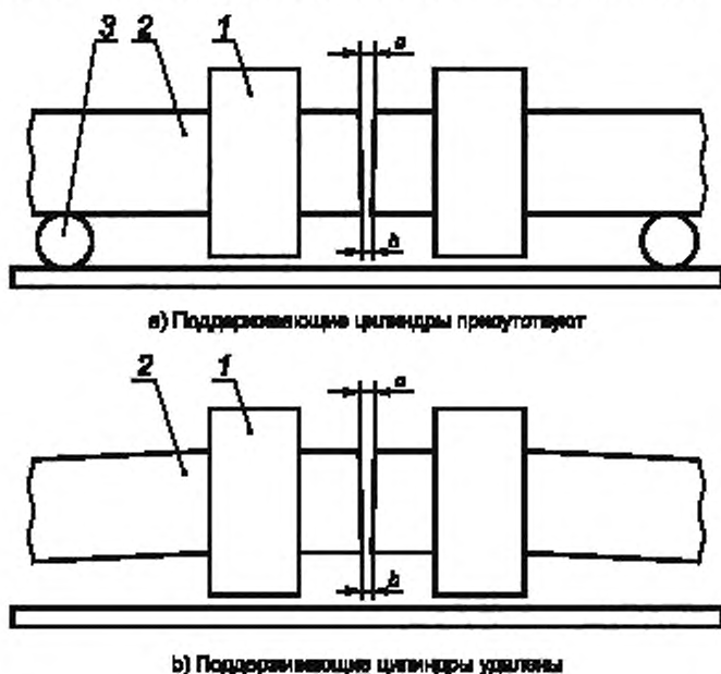
Рисунок 1 — Зазор между трубами при изгибе
