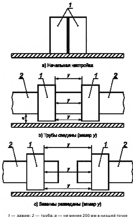
Рисунок 4 — Испытания на подтверждение центрирующей способности зажимов
