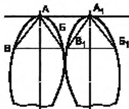
Рисунок 6 — Измерение симметричности носков
