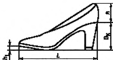
Рисунок 3 — Измерение высоты, длины полуботинок, туфель, высоты каблука и приподнятости носочной части
