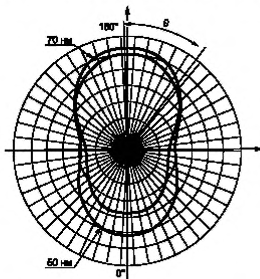
Рисунок 1 — Пример индикатрисы рассеяния для наночастиц размерами 50 и 70 нм на длине волны 405 нм
