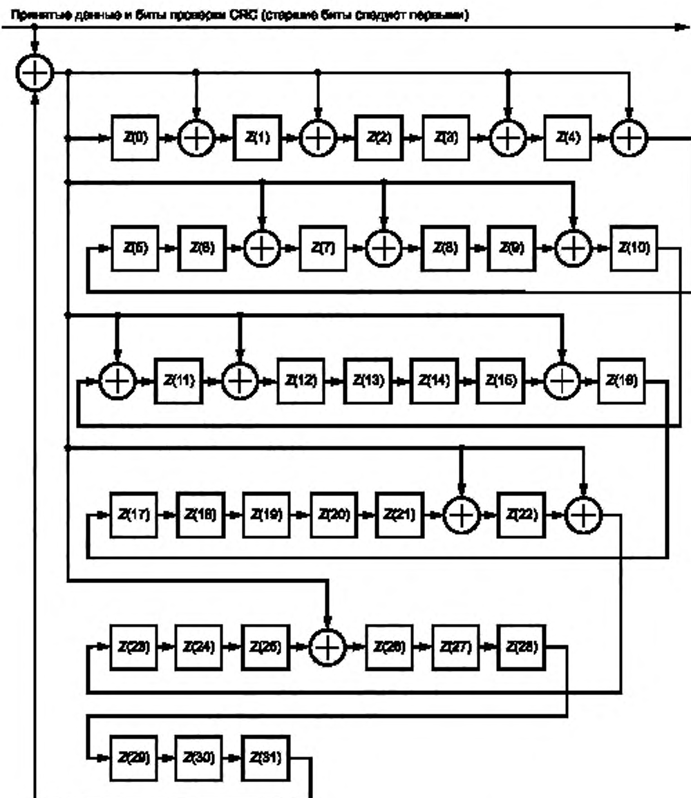
Рисунок А.1 — Модель декодера CRC-32
