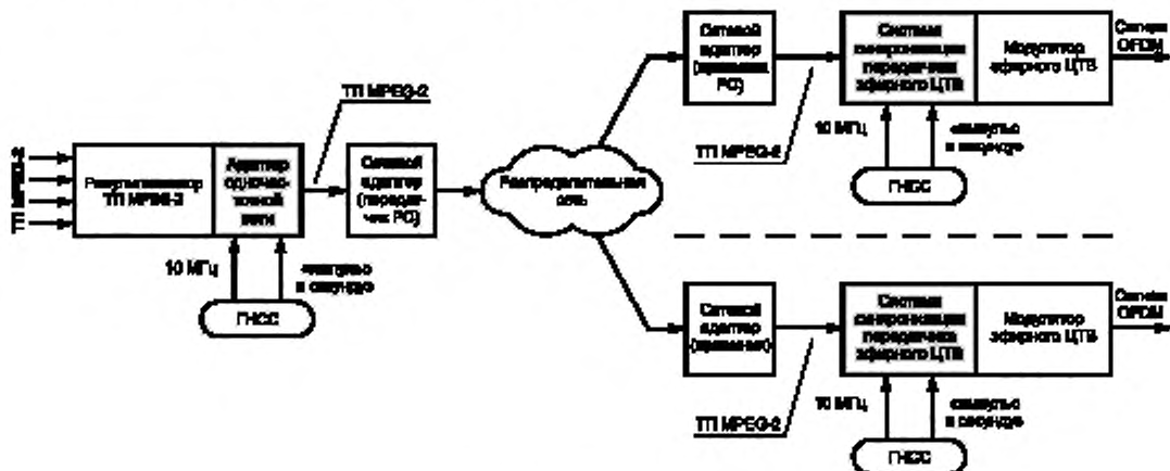
Рисунок 1 — Структурная схема ОЧС
