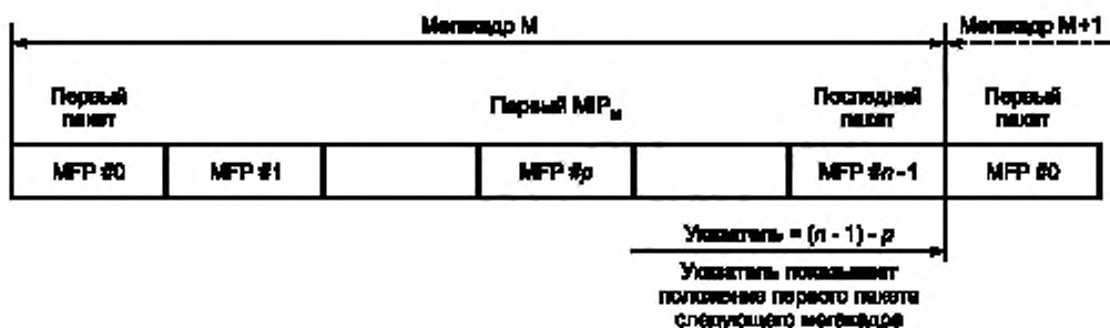
Рисунок 2 — Общая структура мегакадра
