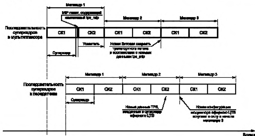
Рисунок В.1 — Процесс изменения конфигурации параметров модулятора эфирного ЦТВ при помощи MIP-пакетов
