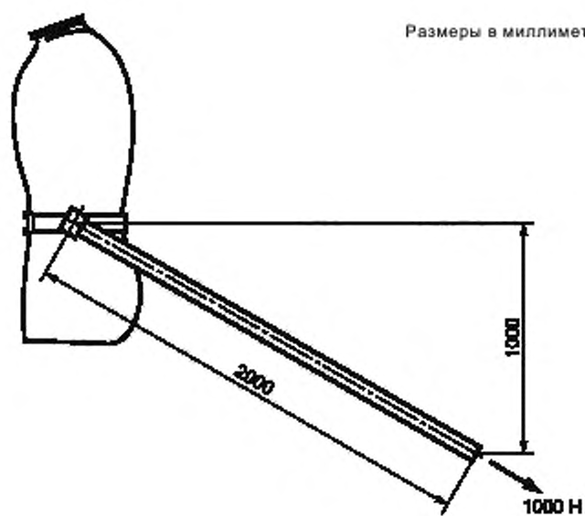
Рисунок 2 — Устройство для испытания прочности пояса или ремня шланга подачи сжатого воздуха и разъемов
