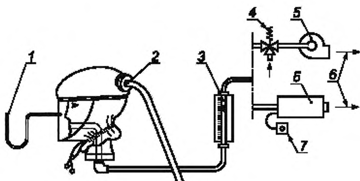
1 — микроанометр; 2 — соединительный шланг низкого давления; 3 — расходомер; 4 — регулятор подачи; 5 — побудитель расхода; 6 — выход; 7 — регулятор подачи
