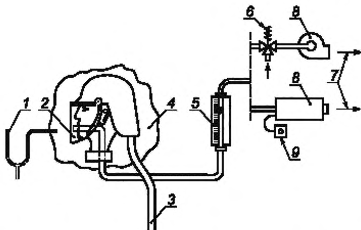
1 — микроанометр; 2 — неплотно прилегающая лицевая часть, 3 — соединительный шланг низкого давления; 4 — легкий пластиковый пакет; 5 — расходомер; 6 — регулятор подачи; 7 — выход; 8 — всасывающее устройство; 9 — регулятор подачи
