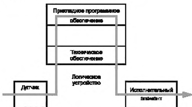
Рисунок С.1 — Логическое решающее устройство
