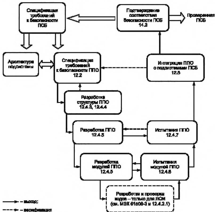
Рисунок 3 — Жизненный цикл разработки ПО (V-модель)
