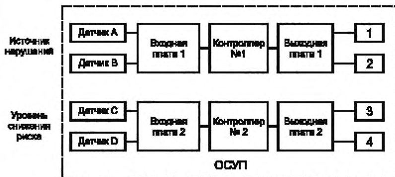
Рисунок 2 — Функция ОСУП и независимость источника нарушений
