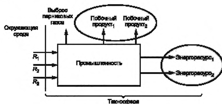
Рисунок 3 — Многовыходная система
