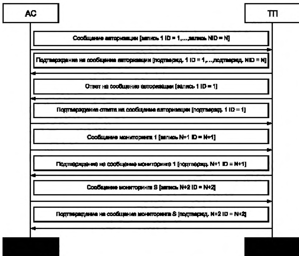
Рисунок 3 — Диаграмма обмена сообщениями
