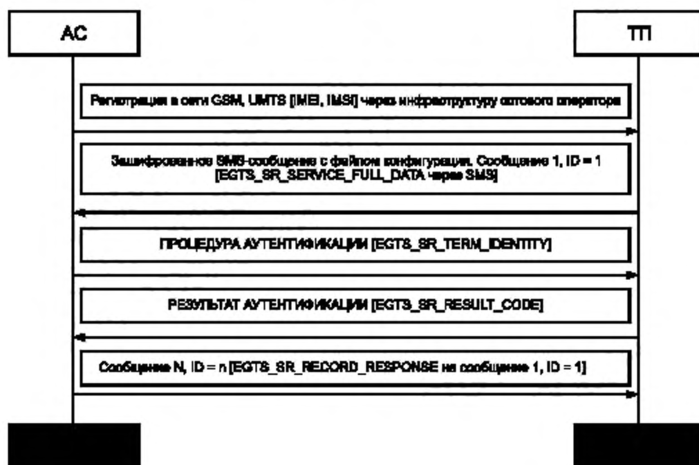
Рисунок 4 — Алгоритм конфигурирования АС с использованием SM
