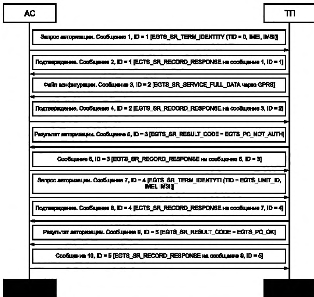
Рисунок 5 — Алгоритм конфигурации AC с использованием GPRS
