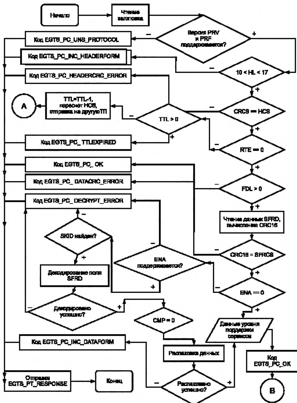
Рисунок 1 — Блок-схема алгоритма сборки пакета протокола транспортного уровня при приеме
