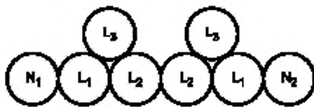
Рисунок Н.52.3 — Специальная конфигурация для шести параллельных одножильных кабелей, уложенных треугольником (см. 523.7)
