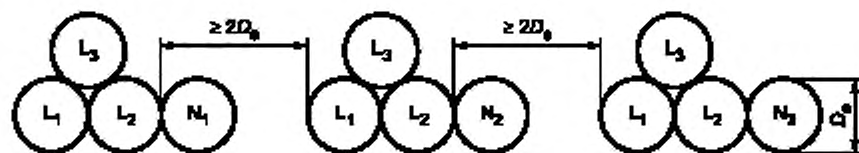
Рисунок Н.52.6 — Специальная конфигурация для девяти параллельных одножильных кабелей, уложенных треугольником (см. 523.7)
