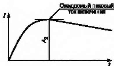
Рисунок 7б — Калибровка испытательной цепи для постоянного тока
