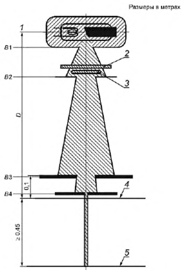
1 — диафрагмы луча излучения ( B_1 , B_2 , B_3 , B_4 ); 2 — дополнительный фильтр; 3 — контрольный детектор ( R_1 ); 4 — пленка; 5 — ширма из свинца; D — переменное расстояние
