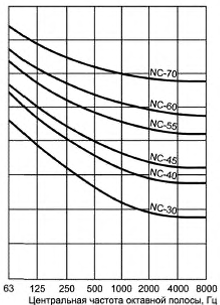
Рисунок 2 — Кривые зависимости критерия (NC) помех для телефонной связи
