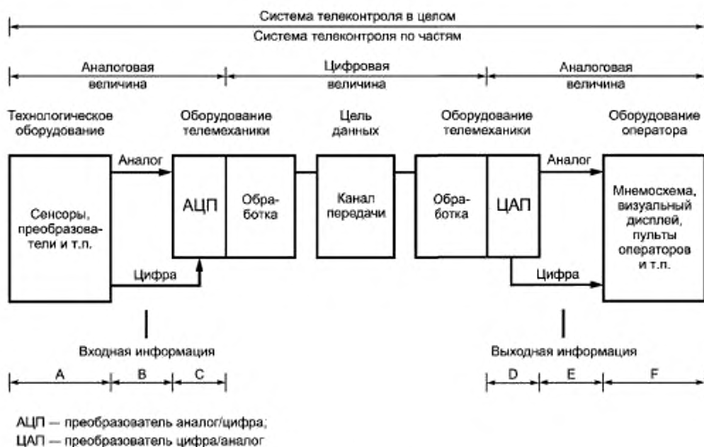
Рисунок 1 — Обработка аналоговой информации
