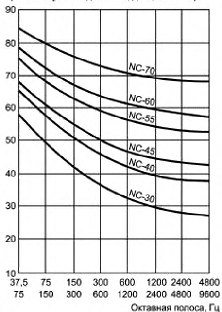
Рисунок 2 — Кривые зависимости критерия (NC) помех для телефонной связи
