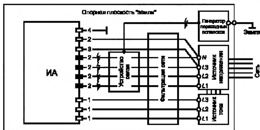
Рисунок Е.2 — Установка для проведения испытаний на устойчивость к наносекундным импульсным помехам. Цели напряжения
