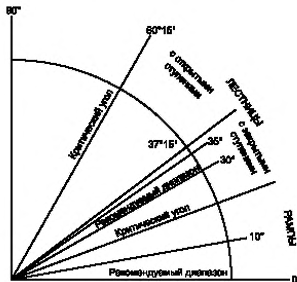
Рисунок 1 — Углы наклона средств доступа к рабочему месту
