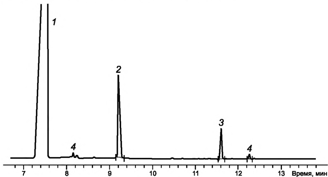
1 — монопентаэритрит; 2 — маннит; 3 — дипентаэритрит; 4 — неидентифицируемые примеси
