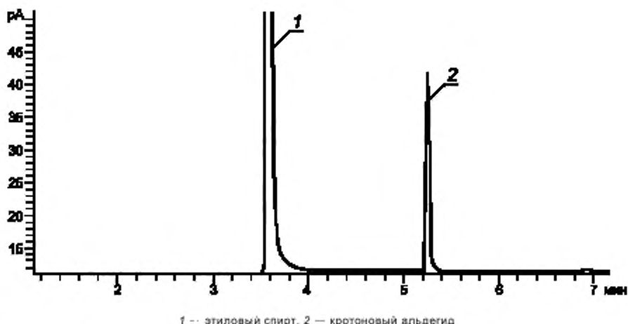
Рисунок 1 — Хроматограмма анализа градуировочной смеси, полученная на хроматографе, оснащённом капиллярной колонкой НР-РРДР*
