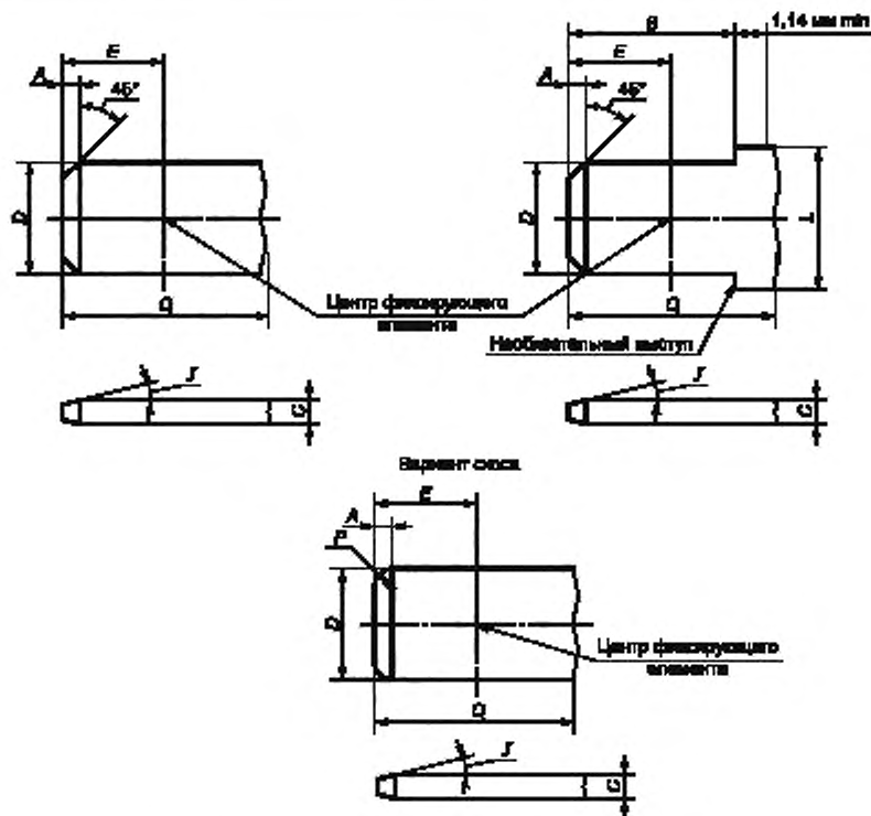
Рисунок 1 — Размеры штыревых контактов (штекеров)
