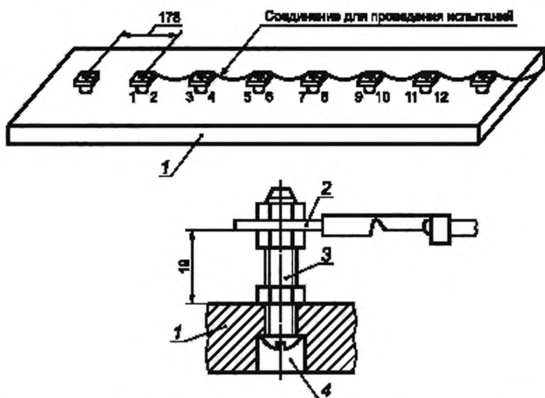
1 — плита из текстолита толщиной 19 мм; 2 — двусторонний штыревой наконечник; 3 — винт и гайка из стали; 4 — цинкованное углубление
