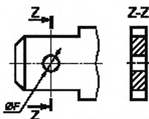
Рисунок 4 — Размеры отверстий для фиксации
