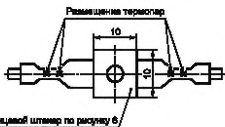
Рисунок 7 — Размещение термодатчиков при испытаниях
