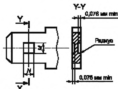
Рисунок 3 — Размеры прямоугольных углублений фиксации
