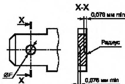
Рисунок 2 — Размеры круглых углублений фиксации (см. рисунок 1)
