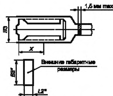
Рисунок 5 — Размеры гнездовых наконечников
