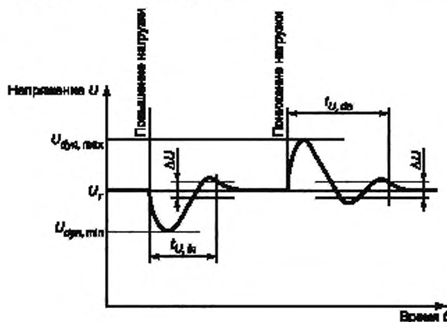
Рисунок 5 — Характеристики кратковременного напряжения без квадратнотокующего статического отклонения напряжения компенсации
