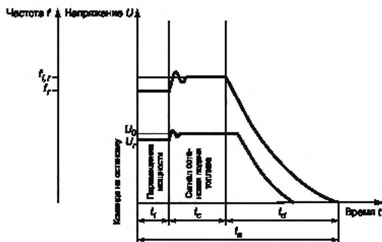
Рисунок 11 — Характеристики остановки
