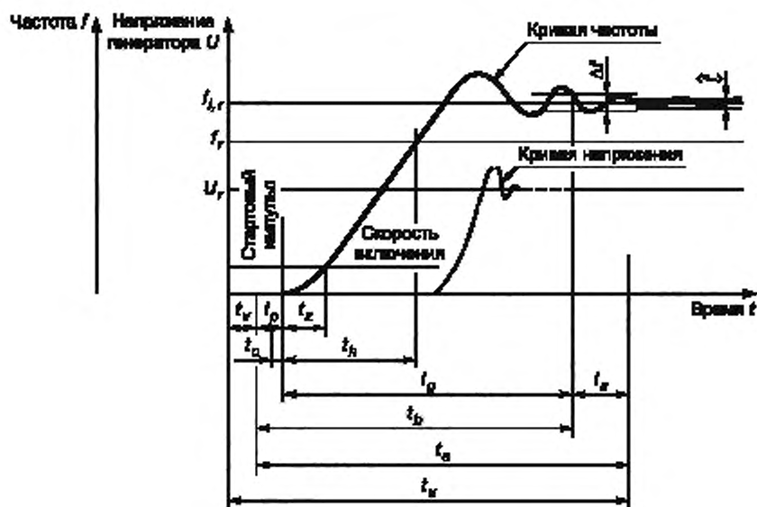
Рисунок 10 — Пусковые характеристики
