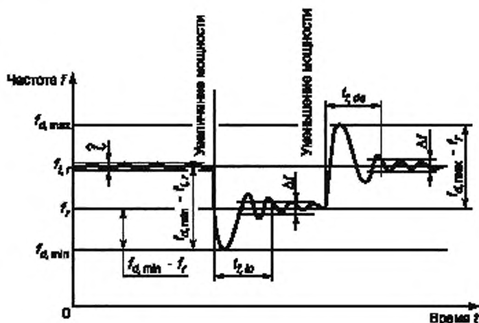
Рисунок 4 — Динамический режим частоты
