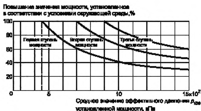
Рисунок 8 — Ориентировочные значения внезапного максимального повышения мощности как функции тормозного эффективного среднего значения давления p_{me} при объявленной мощности (четырёхтактные двигатели)
