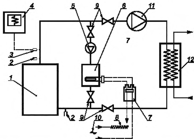
1 — испытуемый котел; 2 — датчики температуры; 3 — низкоинерционная термопара; 4 — самописец; 5 — насос, имеющий такую мощность, что разница температуры между двумя датчиками находится в пределах от 2 °С до 4 °С при максимальной температуре испытаний; 6 — вспомогательный электрический котел; 7 — прибор для измерения электрической мощности; 8 — регулятор напряжения; 9 — клапаны на 1/4 оборота; 10 — электропитание; 11 — дополнительный насос (если требуется); 12 — теплообменник
