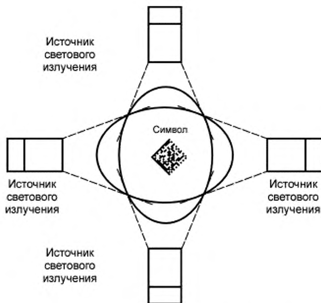
Рисунок 4 — Базовая оптическая схема (вид сверху)
