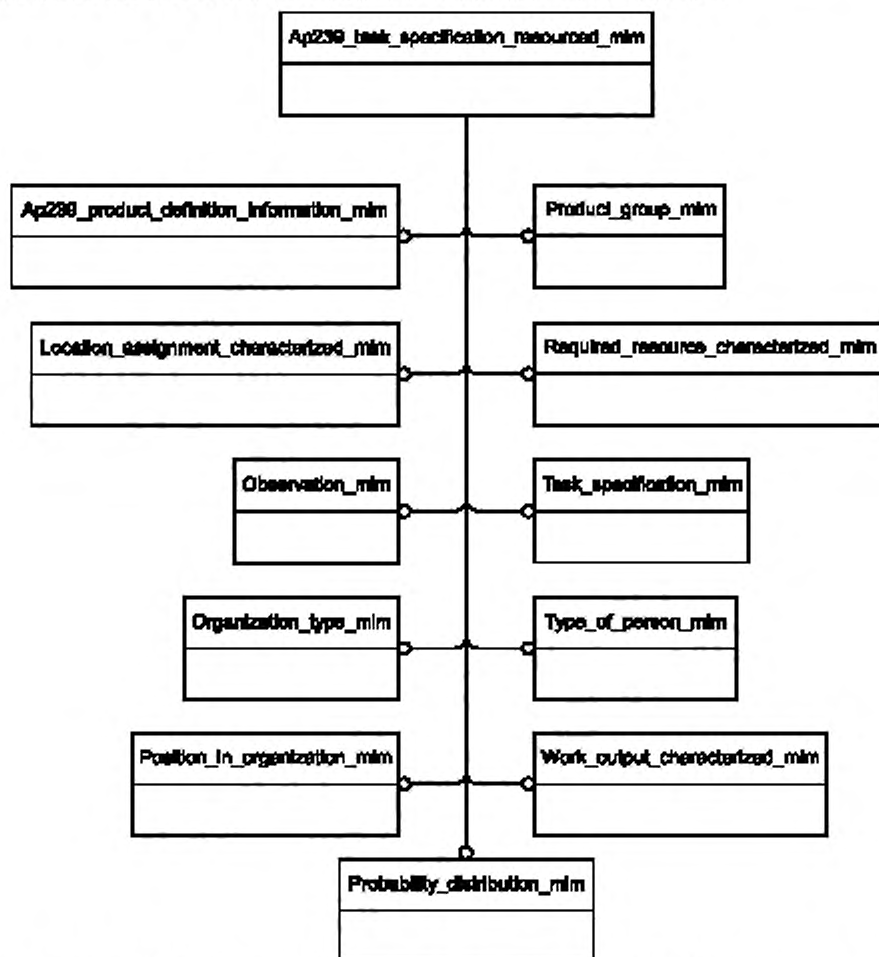
Рисунок D.1 — Представление IMM на уровне схем в формате EXPRESS-G (диаграмма 1 из 1)
