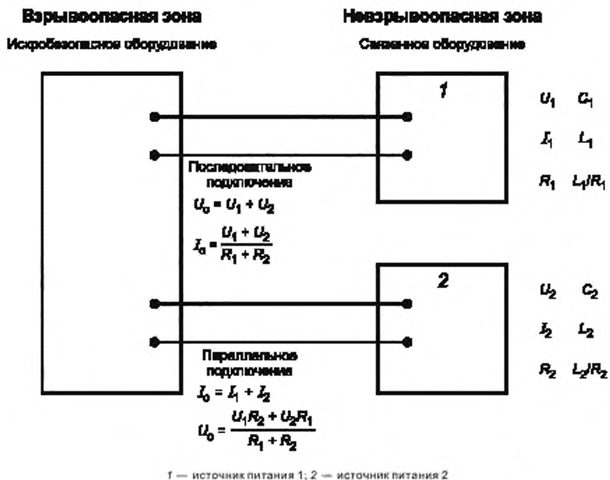
Рисунок В.3 — Произвольно подключенные источники питания
