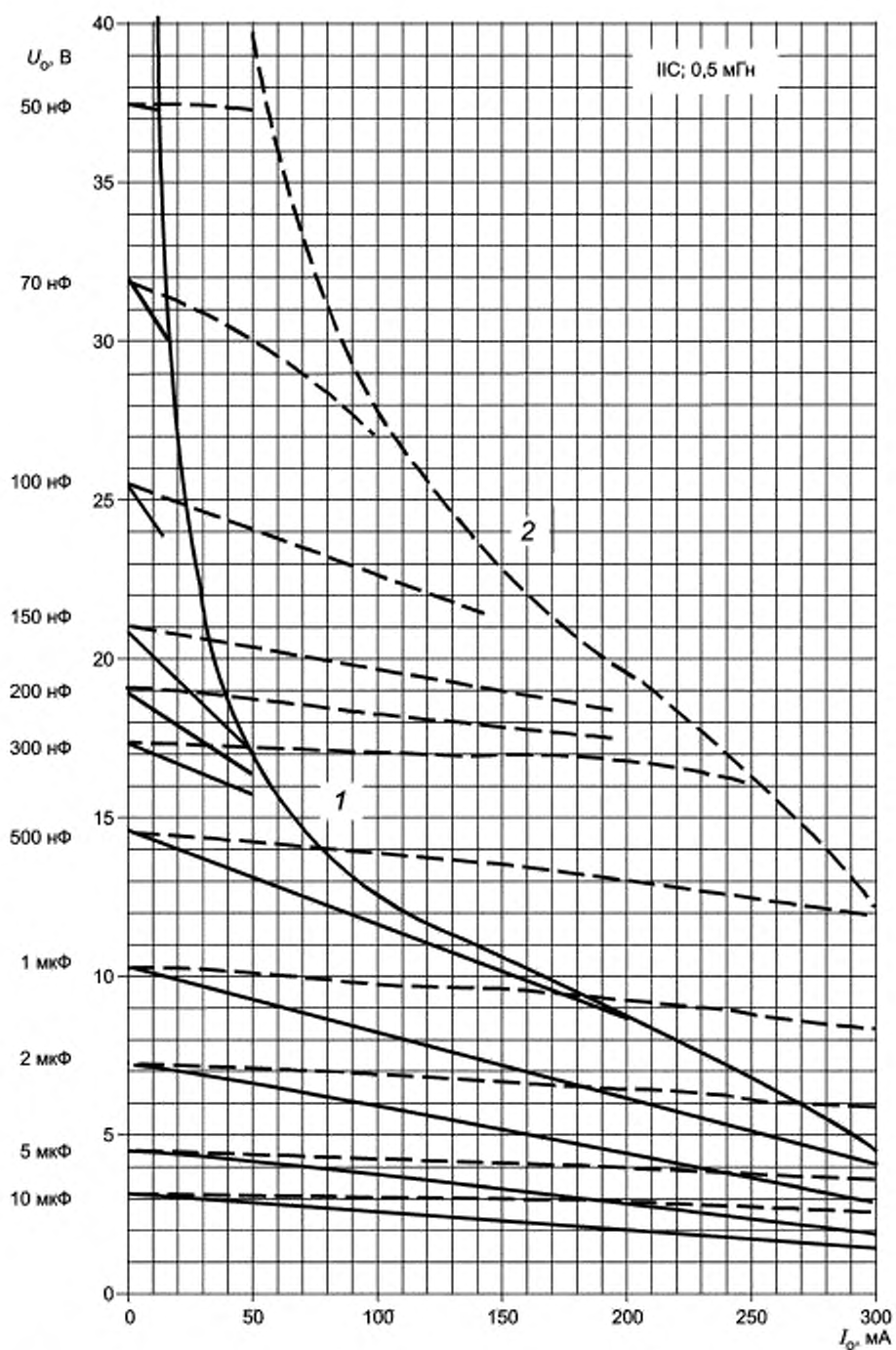
Рисунок С.7б — Диаграмма для значения 0,5 мГн
