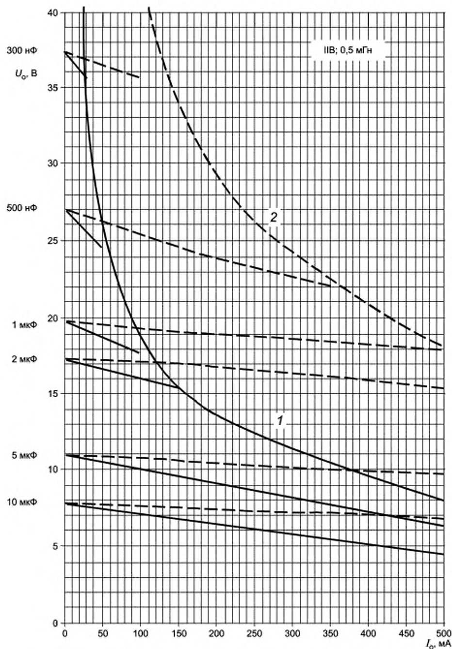
Рисунок С.8в — Диаграмма для значения 0,5 мГн
