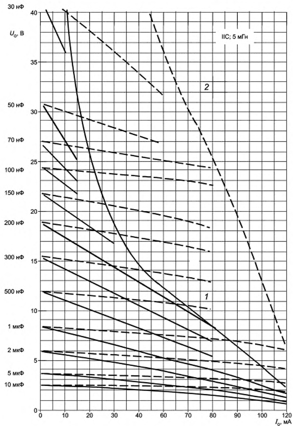
1 — максимальная индуктивность для источника с прямоугольной характеристикой. 2 — максимальная индуктивность для источника с линейной характеристикой
