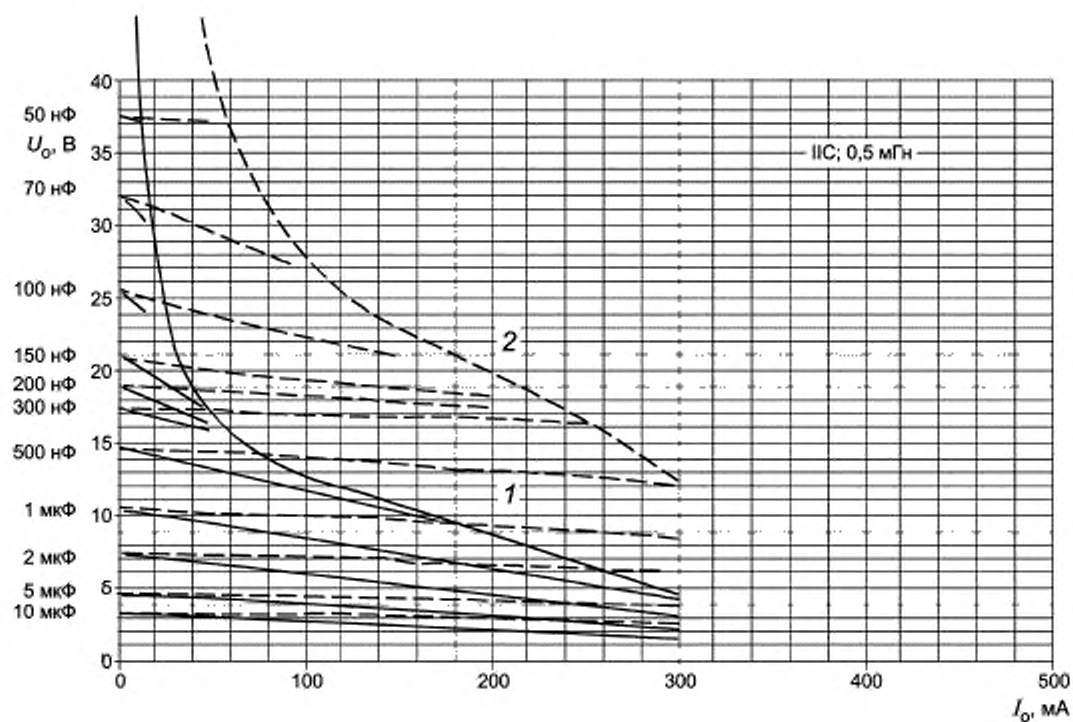
Рисунок С.7б — Диаграмма для значения 0,5 мГн (продолжение)
