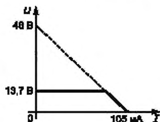
Рисунок С.3а — Выходные характеристики
