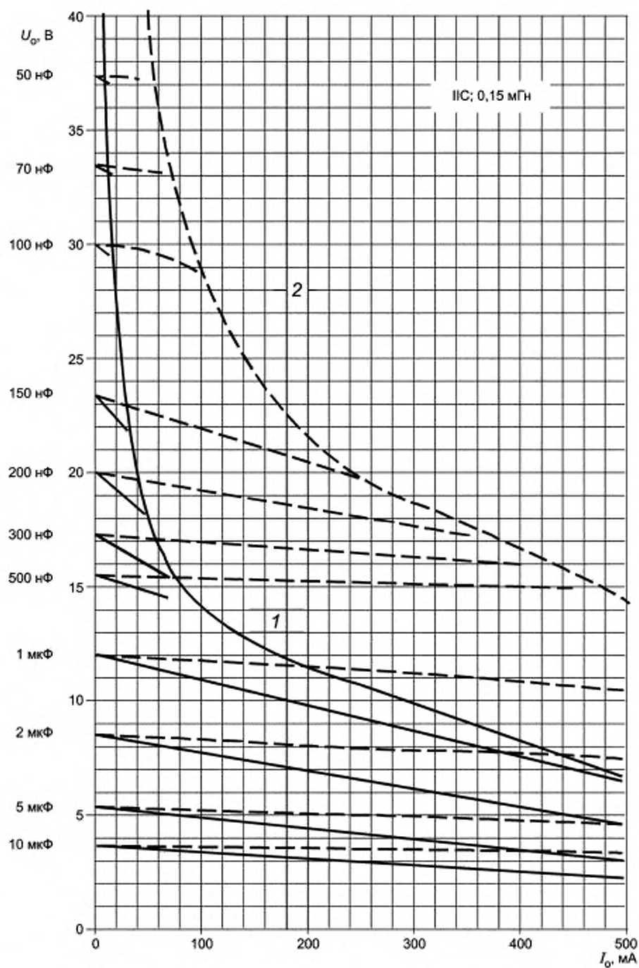
Рисунок С.7а — Диаграмма для значения 0,15 мГн
