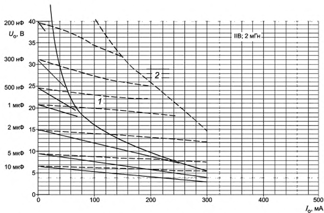
Рисунок С.8d — Диаграмма для значения 2 мГн (продолжение)
