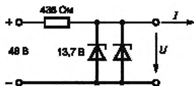
Рисунок С.3б — Эквивалентная цепь
