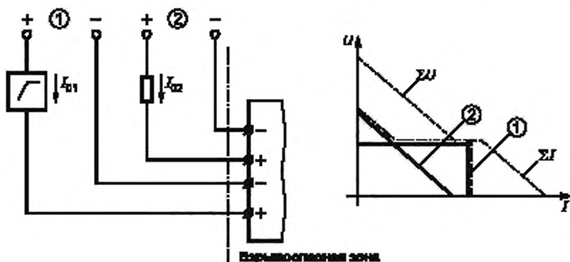
Рисунок С.2е — Последовательное или параллельное подключение со сложением значений тока и напряжения
