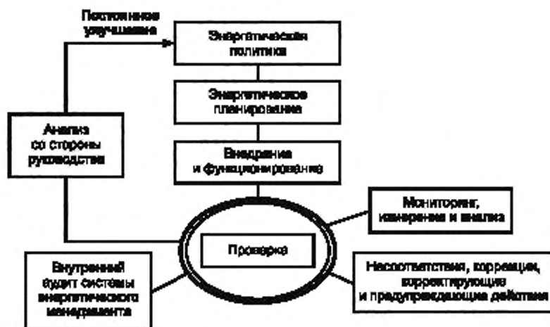
Рисунок 1 — Модель системы энергетического менеджмента для настоящего стандарта
