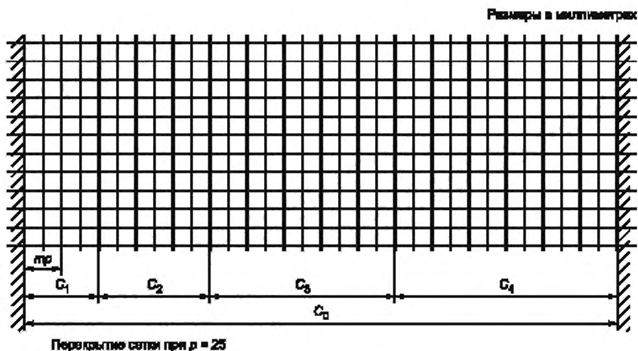
Рисунок 15 — Разделение координационного размера C_0 с помощью одного монтажного шага mp
