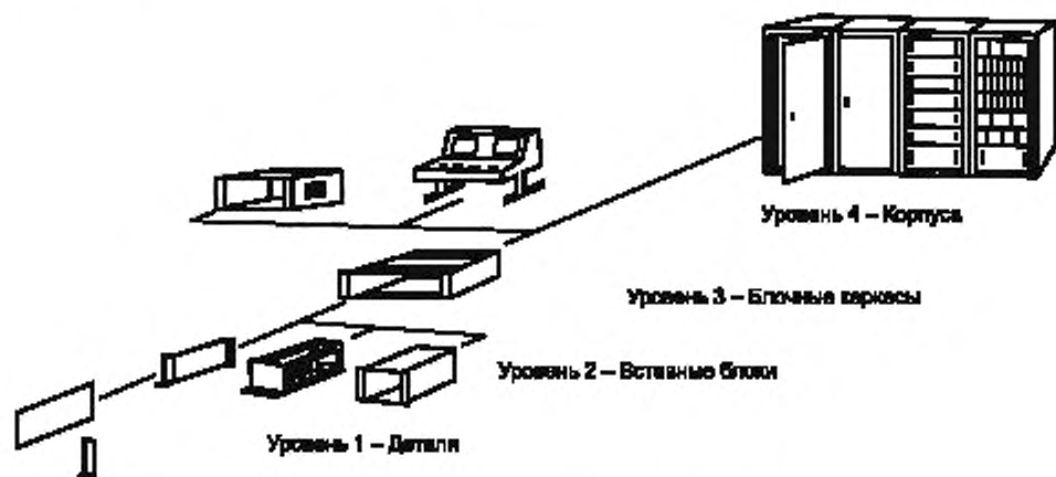
Рисунок 12 — Уровни исполнения несущих конструкций для электронного оборудования 1)
