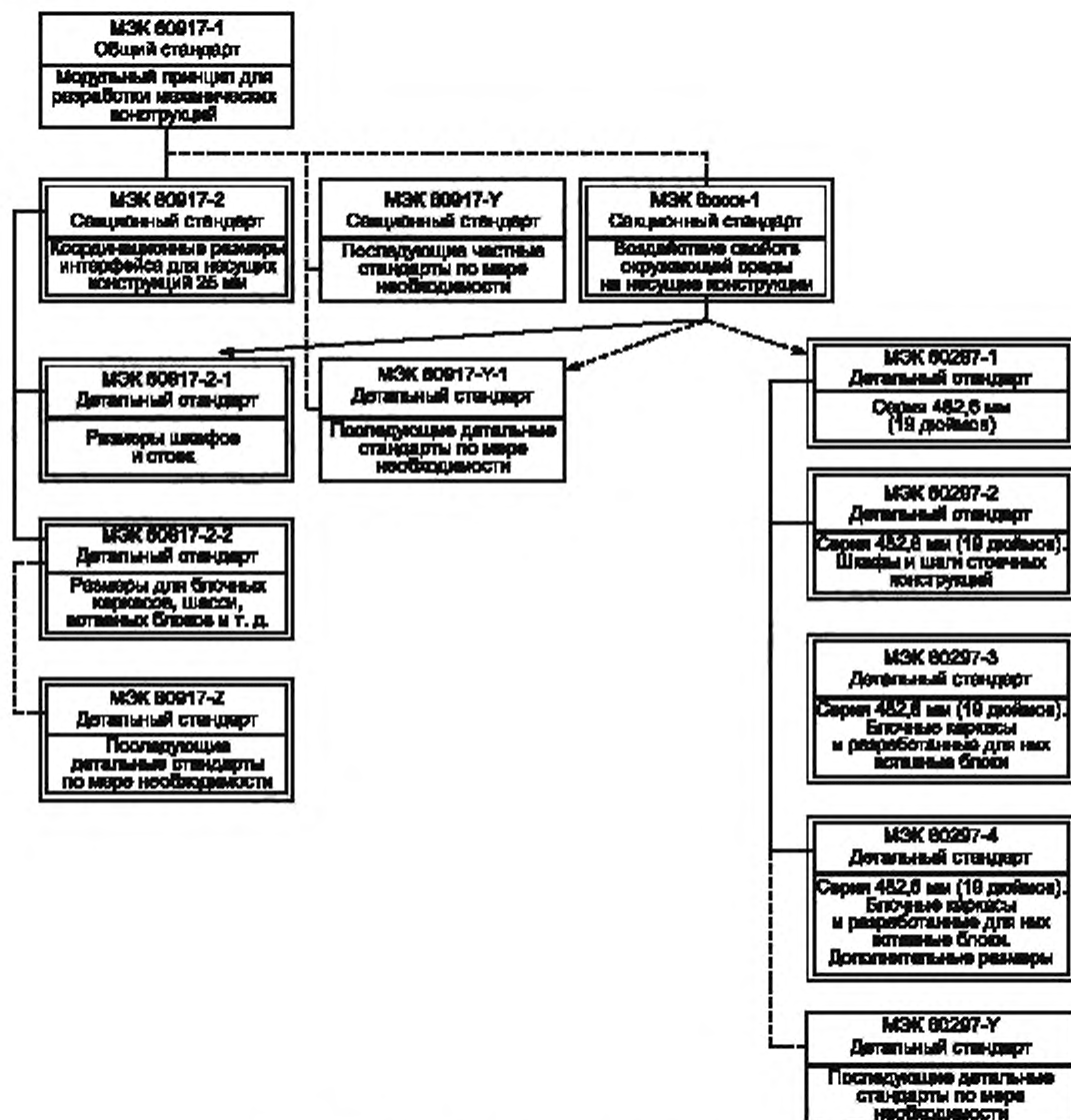
Рисунок 13 — Структура стандартов на несущие конструкции
