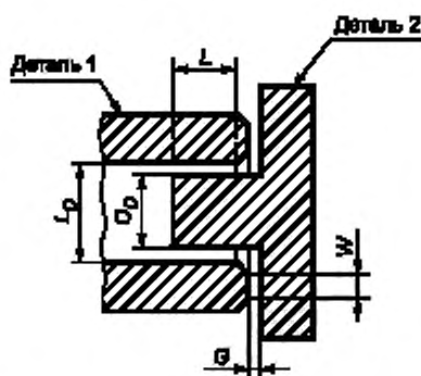
Рисунок 3 — Цилиндрическое соединение
