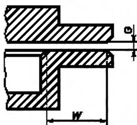
Рисунок 2 — Плоское соединение
