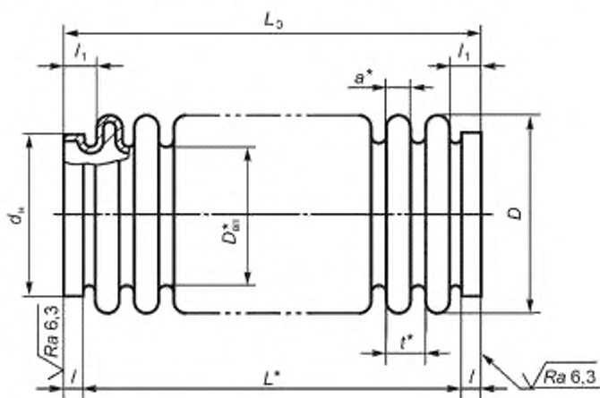
Рисунок 1 — Сиффон многослойный металлический
