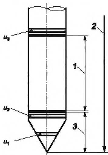
1 — муфта трения; 2 — наконечник; 3 — конус
