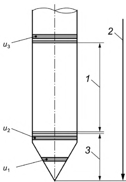
1 — муфта трения; 2 — наконечник; 3 — конус
