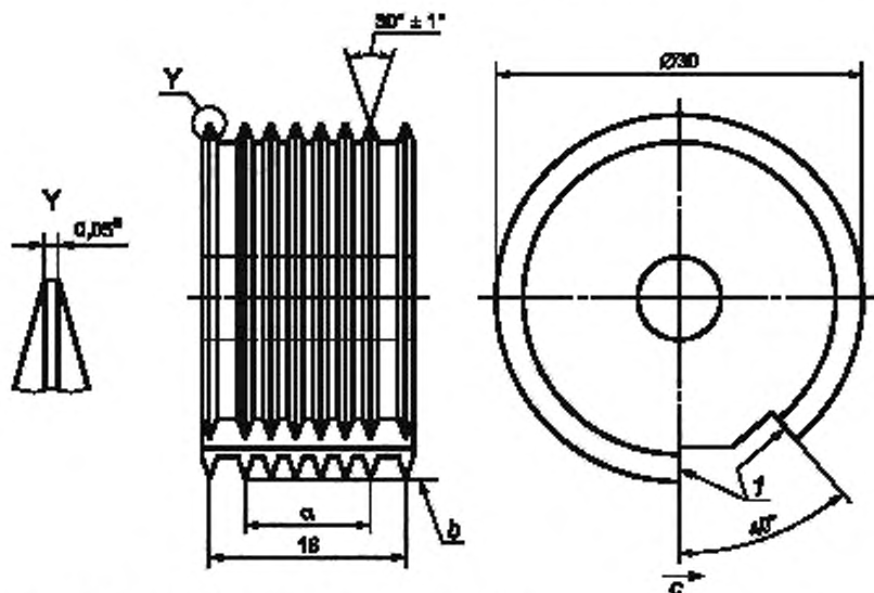
а) Однолезвийный режущий инструмент
