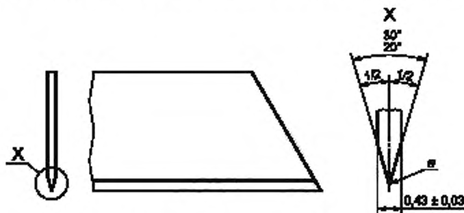
а) Однолезвийный режущий инструмент
