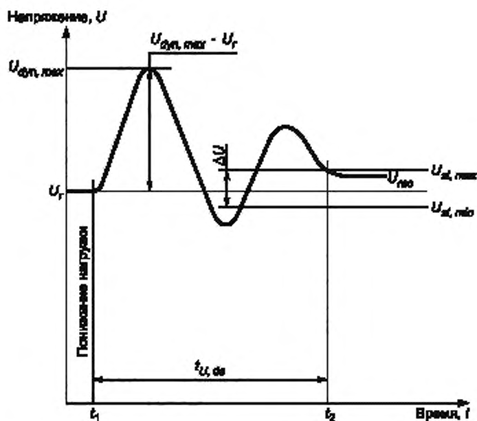
Рисунок А.2 — Характеристика переходного напряжения (понижение нагрузки)
