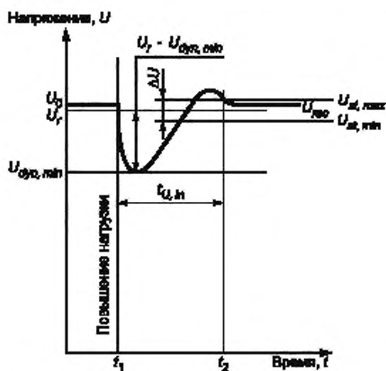
Рисунок А.1 — Характеристика переходного напряжения (повышение нагрузки)
