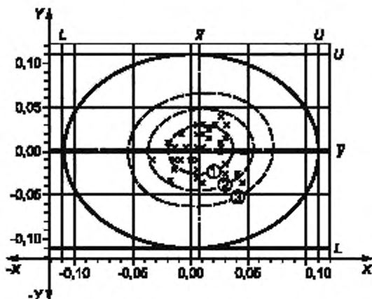
Рисунок 7 — Зона допуска для позиционного допуска
