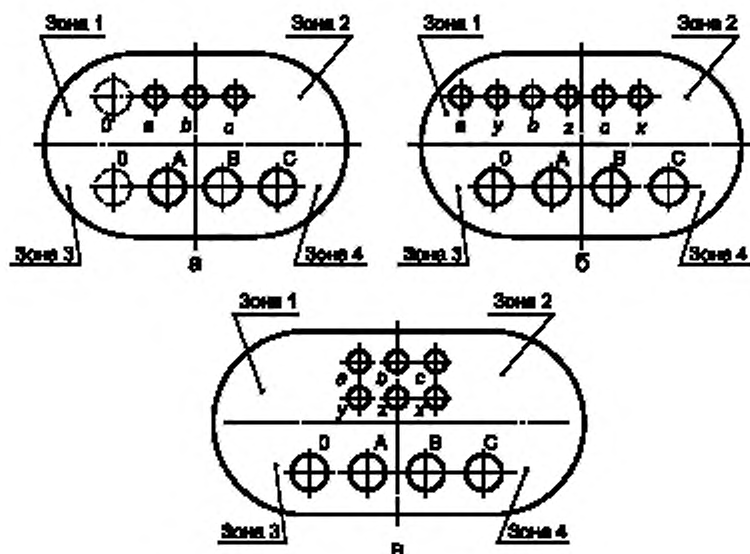
Рисунок 1 — Двухобмоточные трансформаторы
