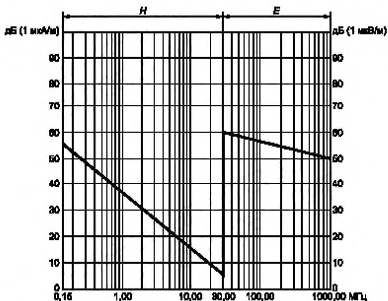
Рисунок 2 — Нормы напряженности поля электромагнитных помех (квасипиковые значения) от тяговых подстанций
