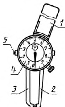
1 — ручка; 2 — неподвижный стержень; 3 — измерительный наконечник; 4 — отчетное устройство; 5 — арретир
