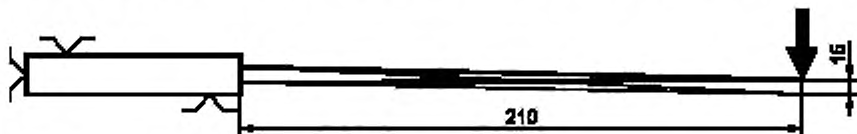
Рисунок 1 — Схема проведения испытания на прочность и упругость охотничьих тесаков
