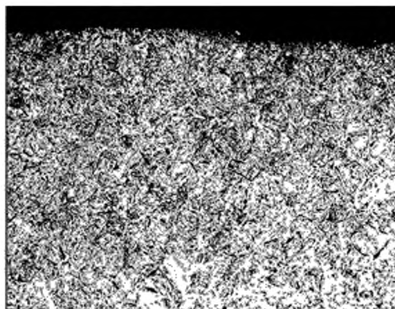
Рисунок 6 — Пример микроструктуры (полностью мартенситной) термообработанной легированной стали, в которой не наблюдаются видимые признаки обезуглероживания (200 \times , травление 2 %-ным спиртовым раствором азотной кислоты)
