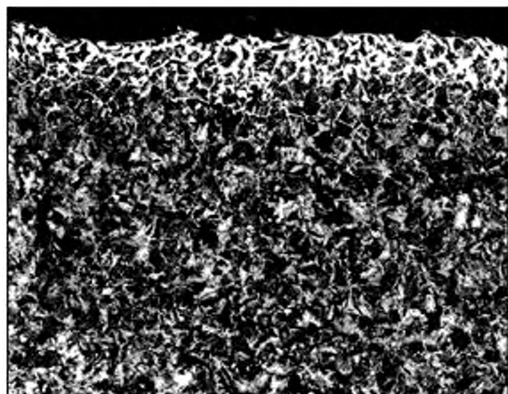
Рисунок 5 — Пример микроструктуры с частичным обезуглероживанием (у поверхности и вблизи нее наблюдается феррит) в полностью перлитной легированной стали в состоянии после прокатки (200 \times , травление 2 %-ным спиртовым раствором азотной кислоты)
