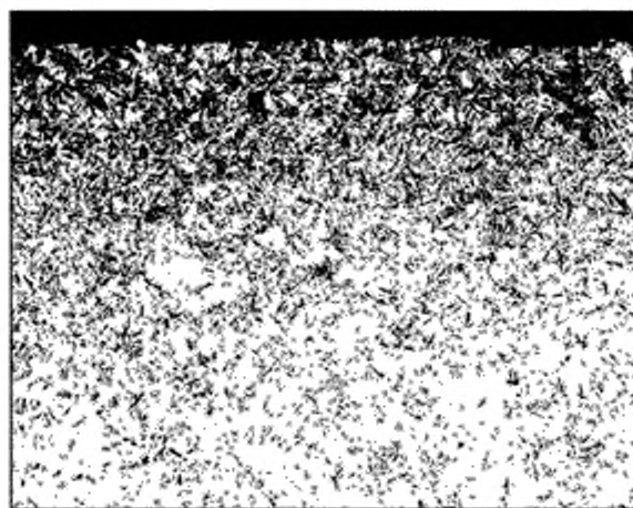
Рисунок 7 — Пример частичного обезуглероживания у поверхности образца термообработанной легированной стали с мартенситной структурой (200 \times , травление 2 %-ным спиртовым раствором азотной кислоты)
