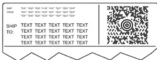
Рисунок A.1 — Размещение символа MaxiCode на этикетке
