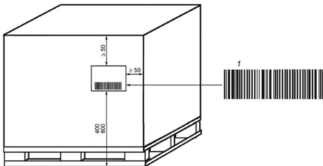
Рисунок 1 — Размещение этикетки на поддоне
