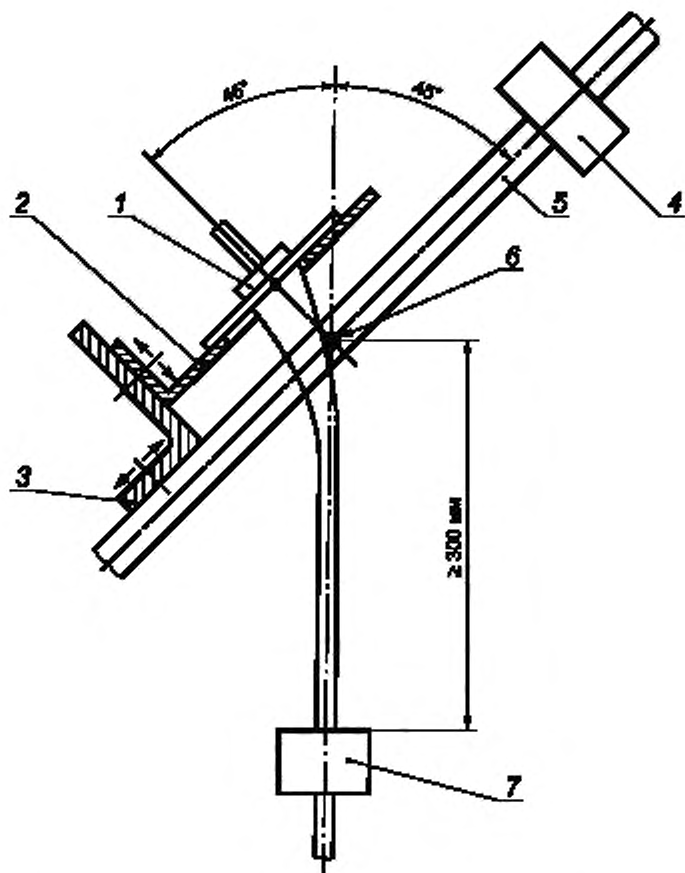
1 – образец; 2 – регулируемая несущая плата; 3 – регулируемый хронштейн; 4 – противовес, 5 – качающаяся рама; 6 – ось качания; 7 – груз
