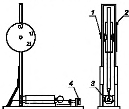
1 – подшипник; 2 – фиксирующийся указатель; 3 – слусовое основание; 4 – слусовой механизм
