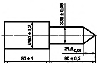
Рисунок 3 – Испытуемый шуп
