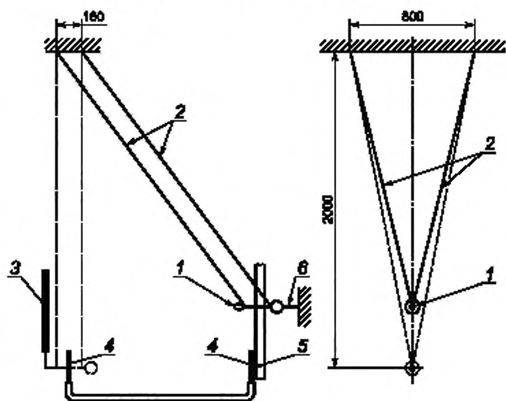
Рисунок R.6 – Установка для настройки калибрующего устройства
