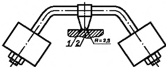
Рисунок 12 – Устройство для вдавливания шарика
