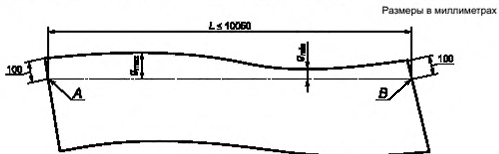
Рисунок 1 — Схема нанесения контрольной линии на полотно материала, длина которого не превышает 10,05 м
