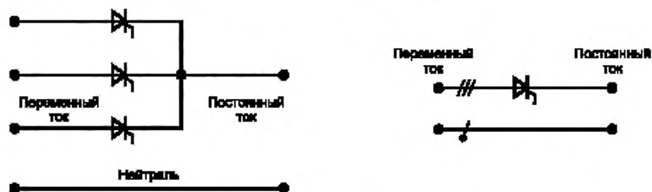
Пример трехфазного преобразователя
