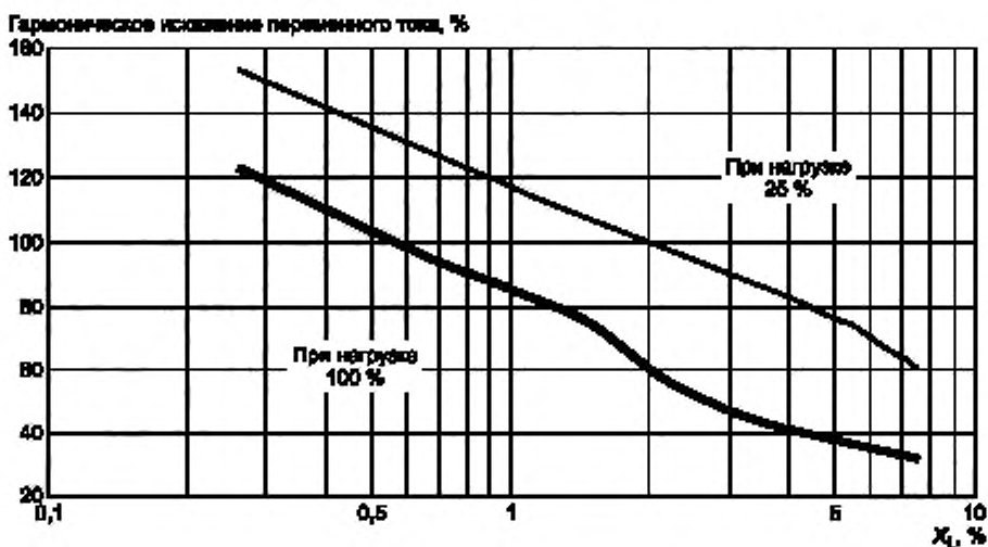
Рисунок В.10 — Искажение входного тока
