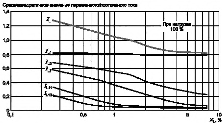
Рисунок В.9 — Входной гармонический ток
