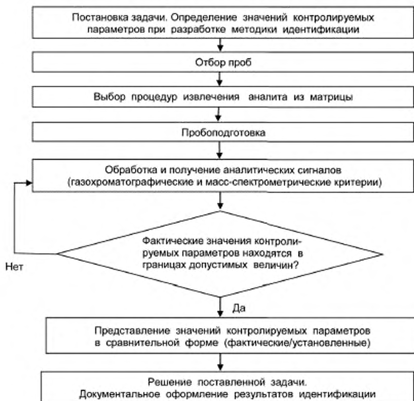
Рисунок 1 — Блок-схема идентификации
