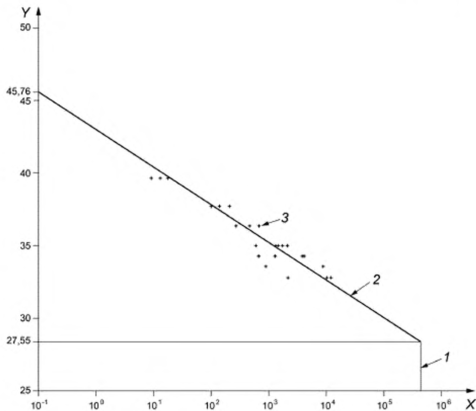
Рисунок А.1 — Линия регрессии, построенная по таблице А.4
