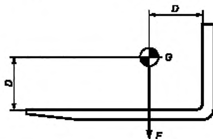
D — расстояние, мм (см. таблицу 2); F — нагрузка; H , G — центр тяжести
