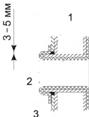
Рисунок 9.8 Пример комбинированного стыкового соединения между футеровками изготовленными различным способом
