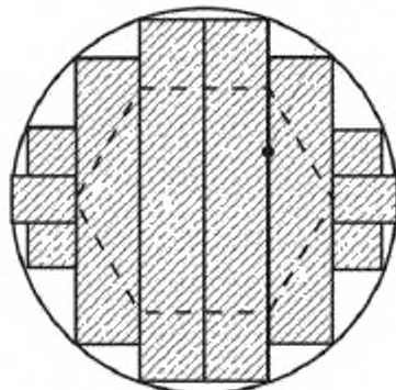
Рисунок А.3 – Раскладка стекляных матов первого слоя
