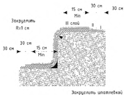
Рисунок 9.1 – Формирование перехода от пола к фундаменту оборудования
