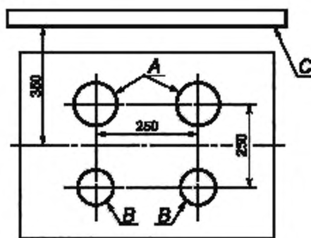
а) Четыре конфорки
