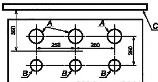
б) Шесть конфорок
