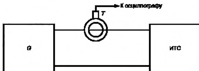
Рисунок А.1 — Схема измерения пикового значения нагрузочного тока ВИ кратковременных прерываний напряжения
