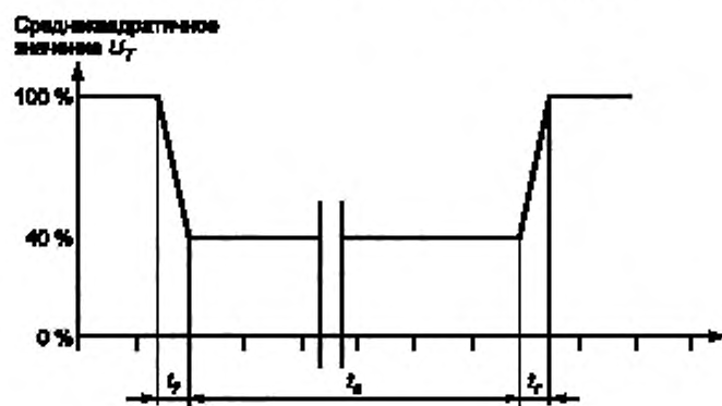
t_p — время нарастания напряжения, t_r — время понижения напряжения; t_s — время выдержки на пониженном напряжении
