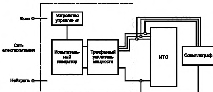
Рисунок С.2 — Схема установки для испытаний трехфазных систем при воздействии провалов, кратковременных прерываний и изменений напряжения электроснабжения
