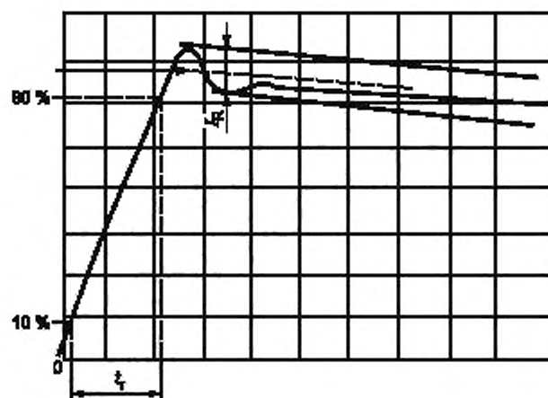
Рисунок 3а — Деление — 50 нс
