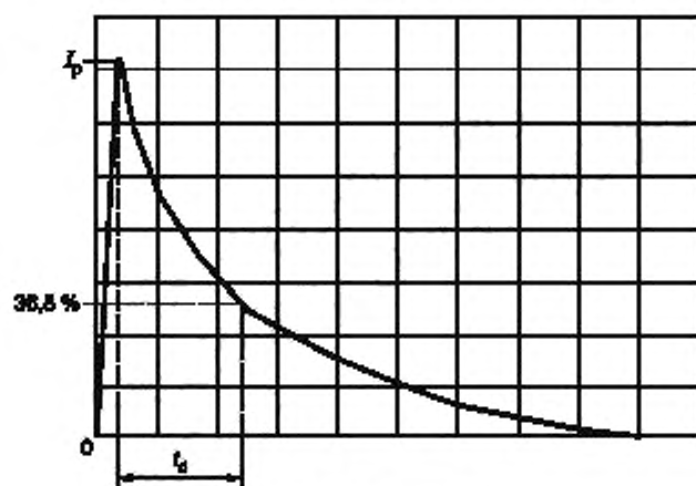
Рисунок 3б — Деление 100 нс
