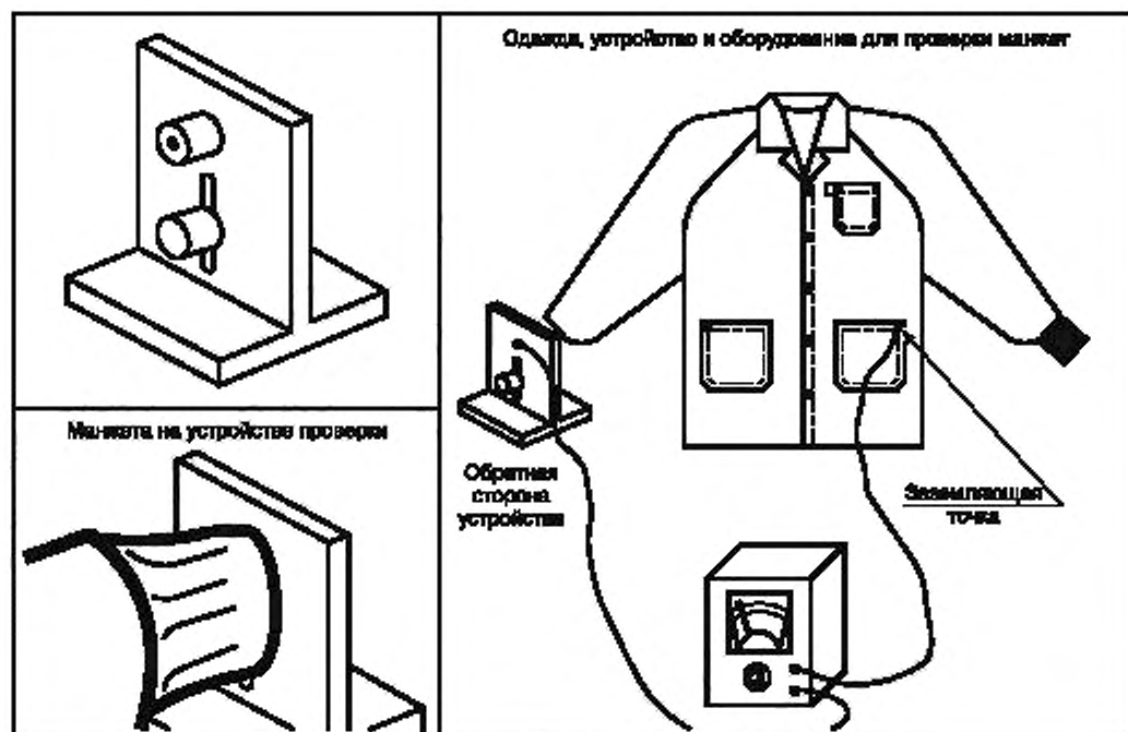
Рисунок 10 — Испытания манжет заземляемой одежды
